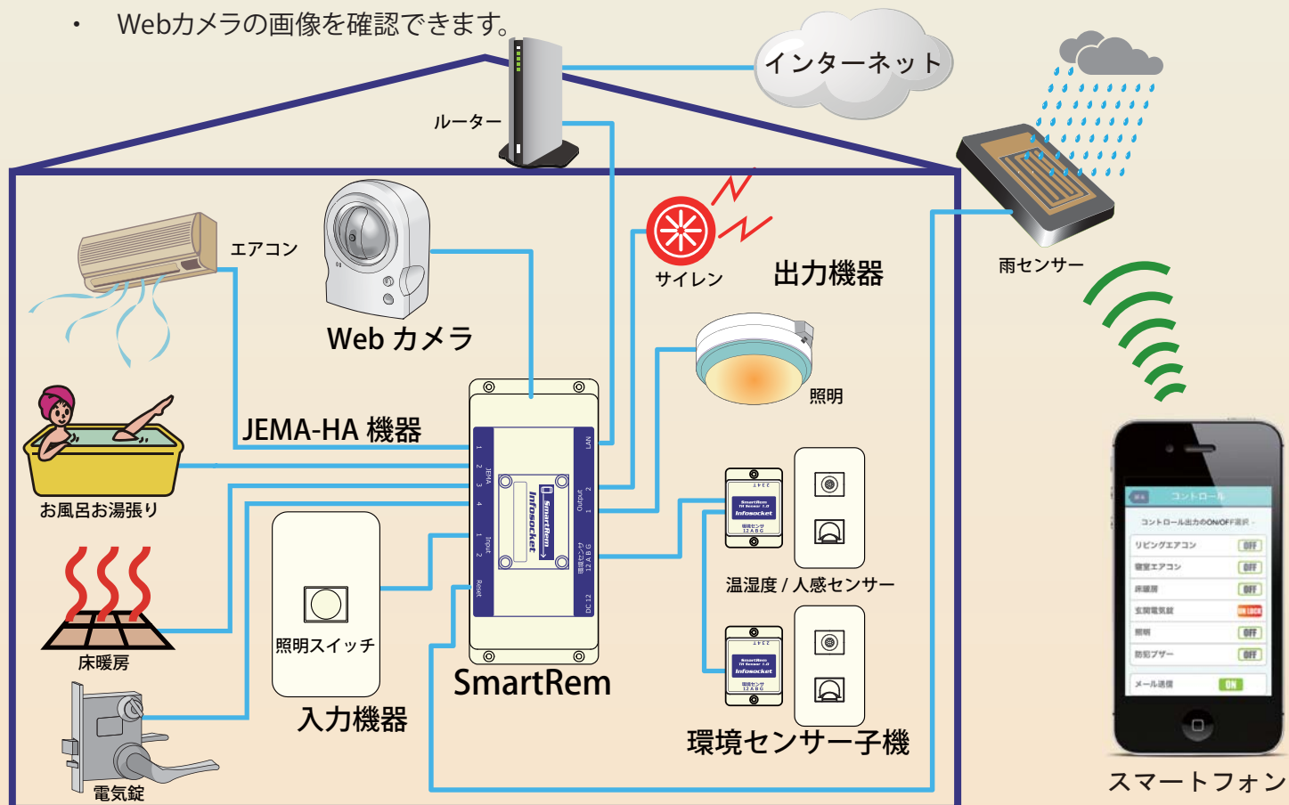
SmartRem システム構成例
